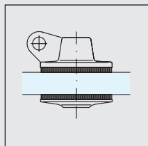
Glasaufhängung
