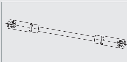
Zugstange je nach Typ M8 / M10 / M12 mit Gabelköpfen
