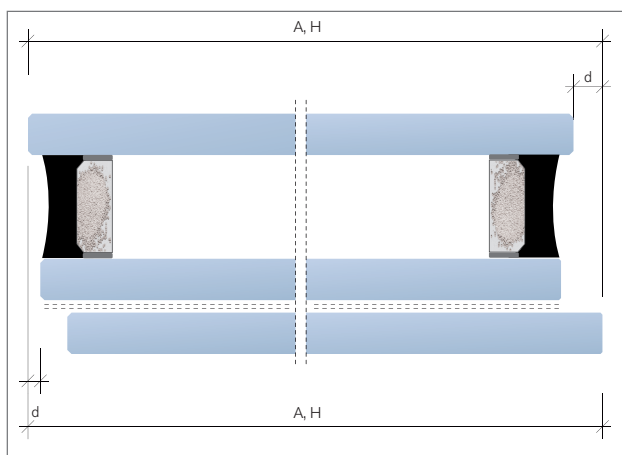
Abb. 29: Kantenversatz bei MIG (d)
