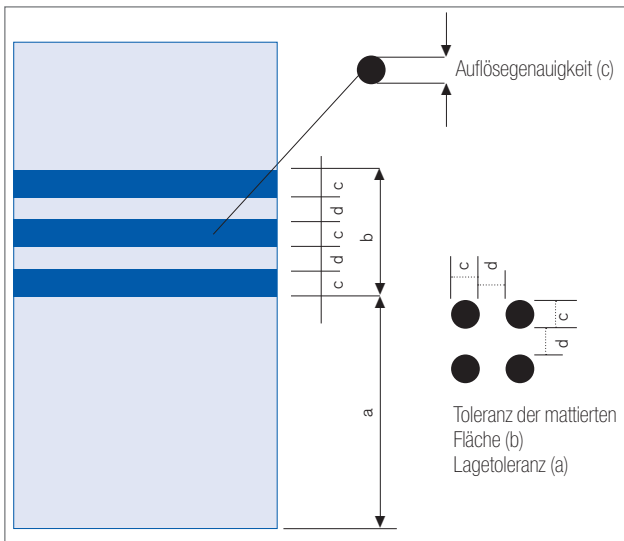
Abb. 19: Geometrie der Abweichung vom Design
