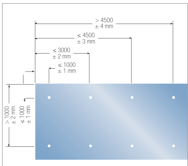
Abb. 14: Lochbohrungslagen
