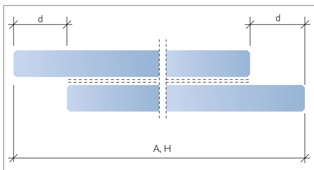
Abb. 29: Kantenversatz bei MIG (d)
