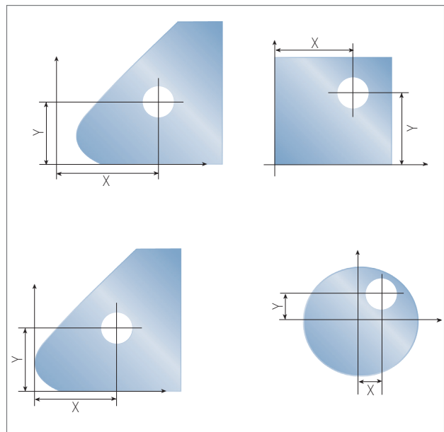
Abb. 13: Bohrlochlage
