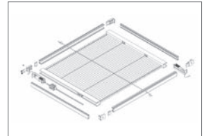
Abb. 6.7: Typ I-Dach
