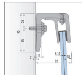
Abb. 8.31: Systemschnitt oben
