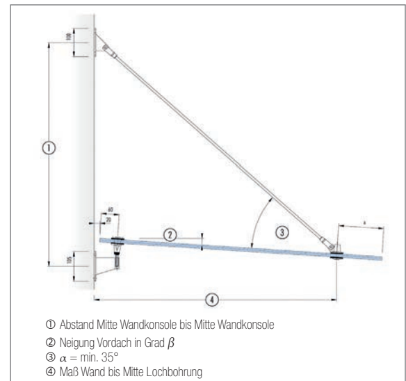
Abb. 8.6: Montageansicht
