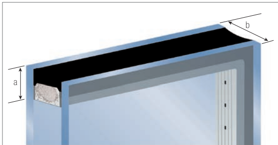
Abb. 10.39: Isolierglas-Randverbund
