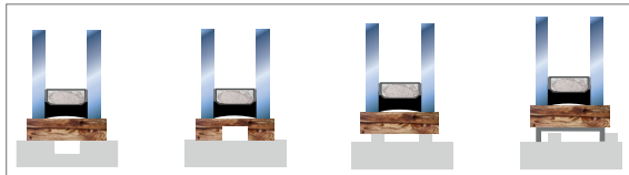
Abb. 10.17: Mögliche Klotzungen
