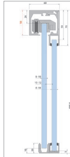
Abb. 8.39: Taschenmontage
