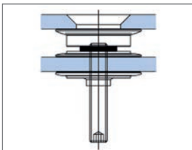
Abb. 8.4: Systemschnitt
