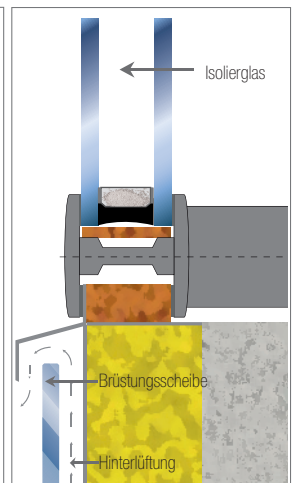
Abb. 6.13: Kalfassade (Systemschnitt)
