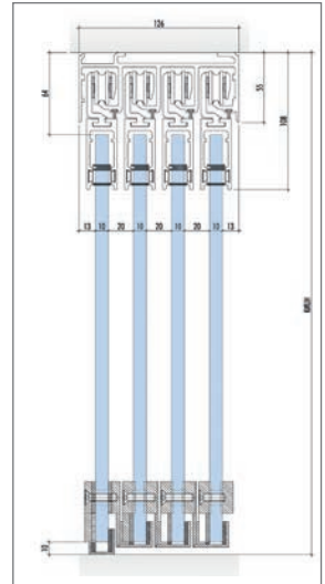
Abb. 8.47: Systemschnitt
