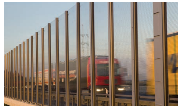
Abb. 5.6: Straßeneinhausung
