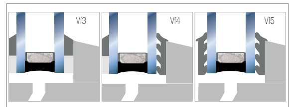
Abb. 10.19: Verglasungssysteme
