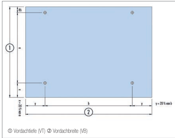
Abb. 8.7: Bohrlochvorlage
