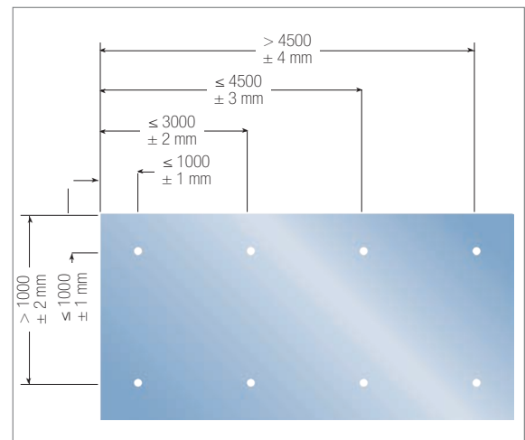
Abb. 10.11: Lochbohrungsanlagen
