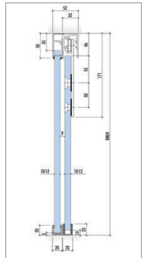
Abb. 8.44: Systemschnitt
