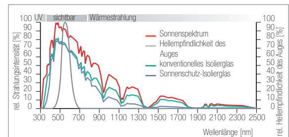
Abb. 3.28: Globalstrahlung
