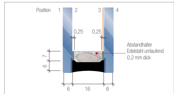
Abb. 3.2: Isolierglas-Aufbau
