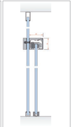
Abb. 8.38: Systemschnitt
