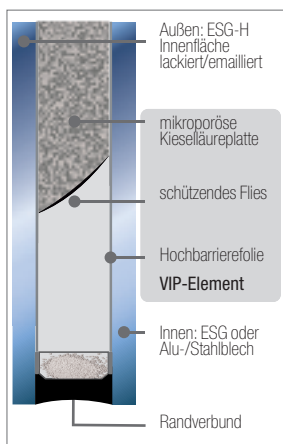
Abb. 4.16: Vakuum-Paneel
