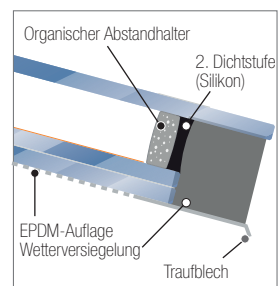
Abb. 10.25: Fehlerhafte Traufpunktversiegelung
