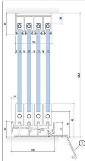
Abb. 8.55: Systemschnitt
